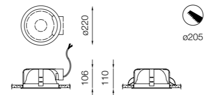
FLC G24q-... round
