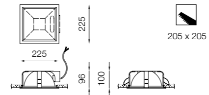
FLC G24q-... square
