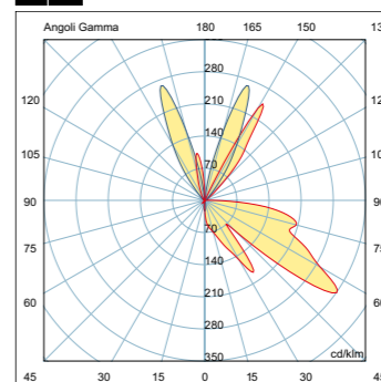
TAM TAM wall reflecta 1x150W
