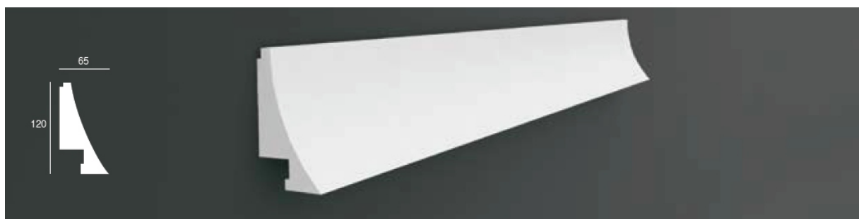
RÉF. 4634 — Vé — Longueur / length 1,20 m
