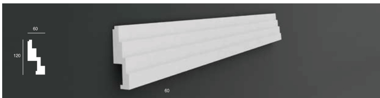
RÉF. 4632 — Crescendo — Longueur / length 1,20 m
