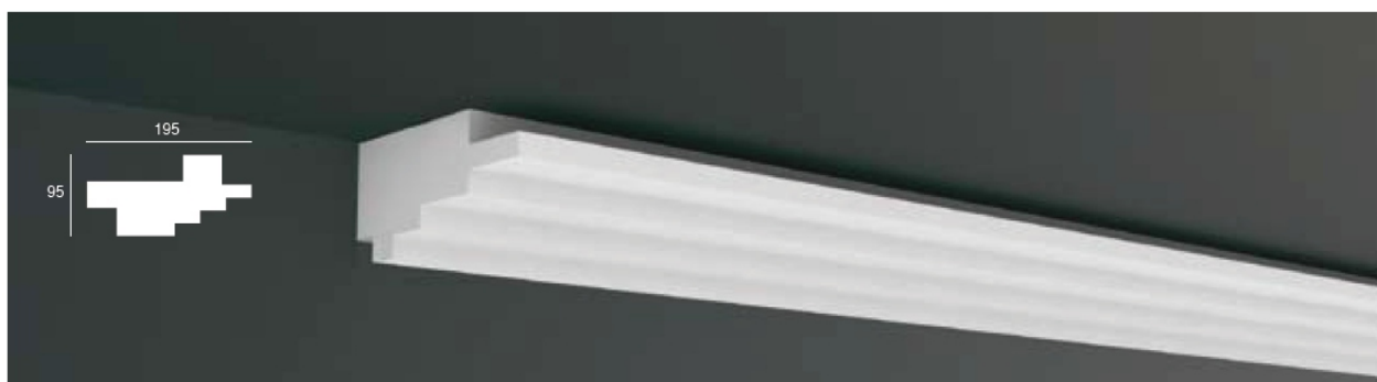
// RÉF. 4622 — Crescendo — Longueur / length 1,20 m
